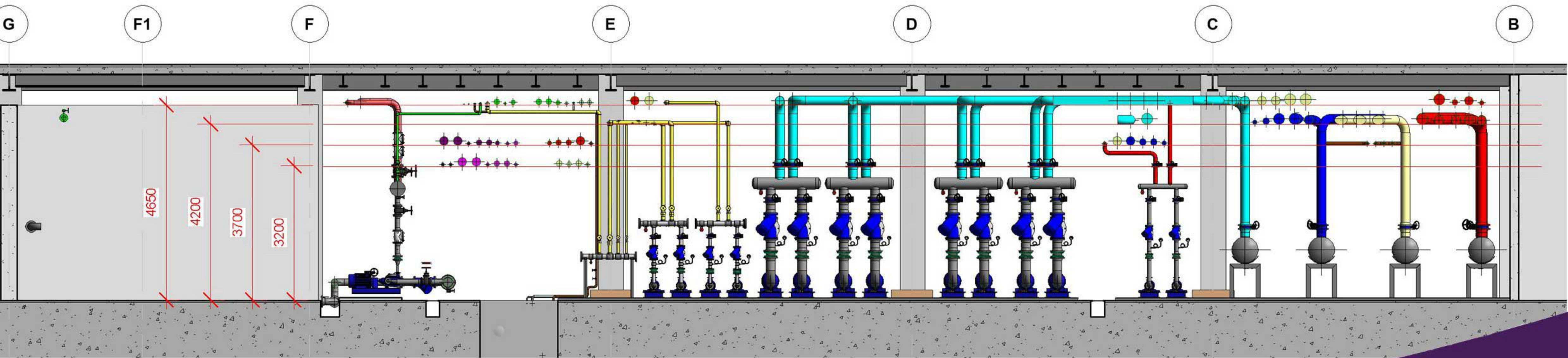
SECTION A-A
